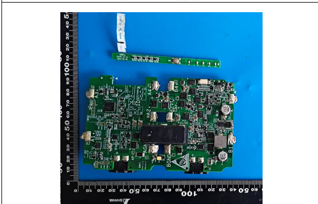
Fig. 5 – Front view of PCM 表5 – PCM 正面视图
