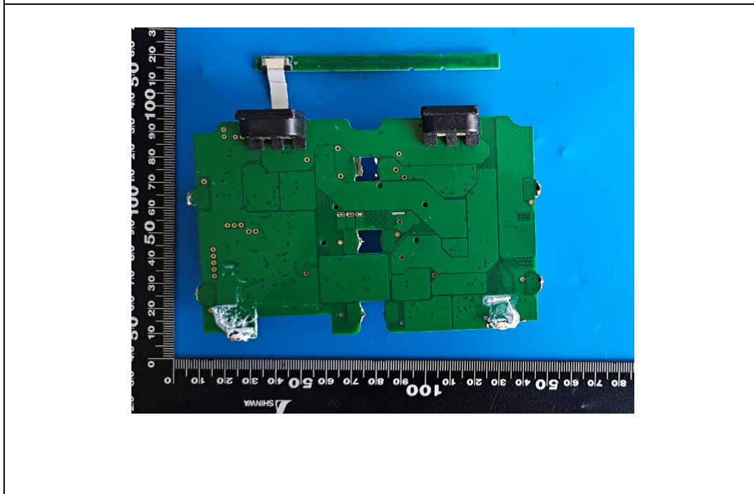
Fig. 6 – Back view of PCM 表6 – PCM 反面视图
